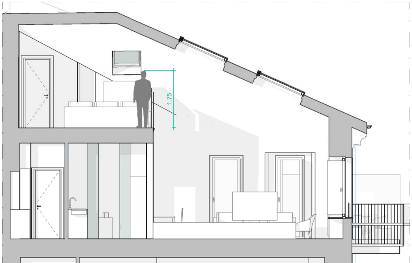
Sezione
