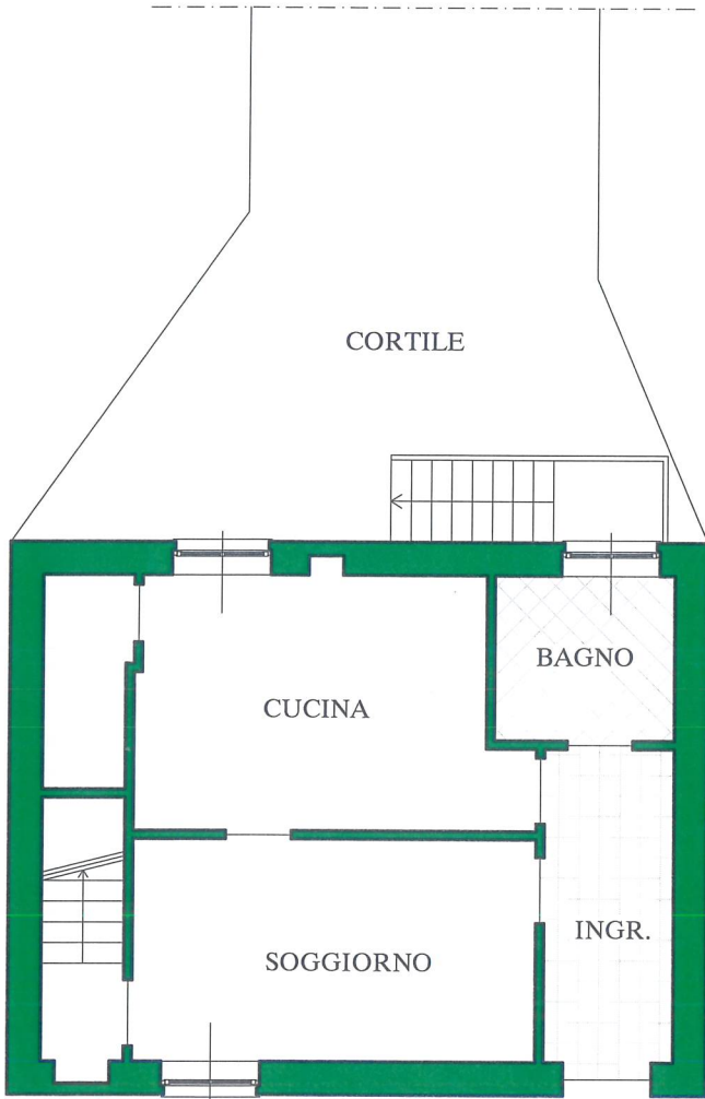
PIANTA P. TERRENO
