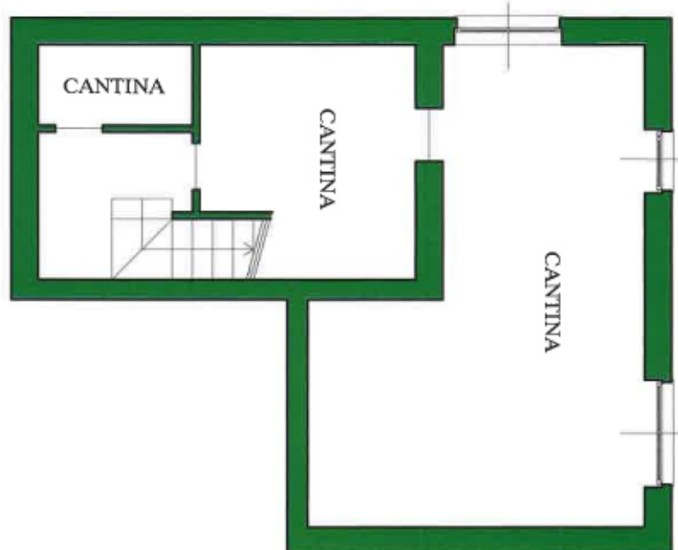
PIANTA PIANO 2° SEMINTERRATO
